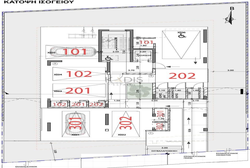
ΚΑΤΟΨΗ ΙΣΟΓΕΙΟΥ
