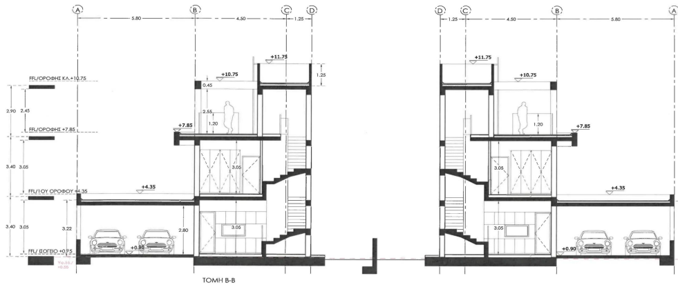
ΤΥΠΟΣ 2 ΚΑΤΟΙΚΙΕΣ Β & Δ
