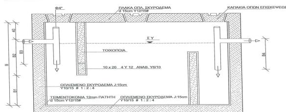
ΤΟΜΗ ΣΥΠΤΙΚΟΥ ΒΟΘΡΟΥ
