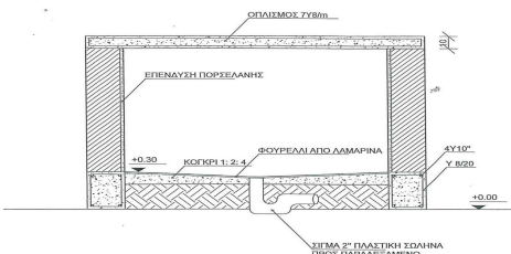
ΤΟΜΗ Β/Β'
