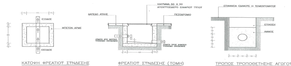
ΚΑΤΟΨΙΣ
