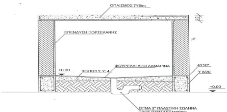
ΤΟΜΗ Β/Β'
