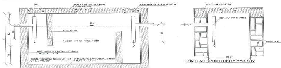
ΤΟΜΗ ΣΥΠΤΙΚΟΥ ΒΟΘΡΟΥ
