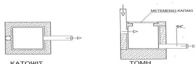
ΦΡΕΑΤΙΑ ΣΥΓΚΕΝΤΡΩΣΕΩΣ
