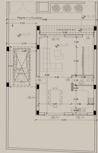
ΚΑΤΟΨΗ ΙΣΟΓΕΙΟΥ
