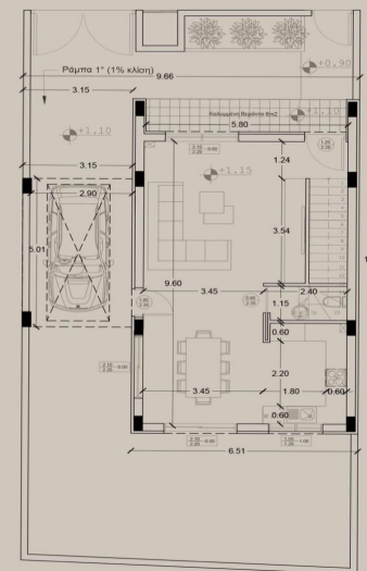
ΚΑΤΟΨΗ ΙΣΟΓΕΙΟΥ
