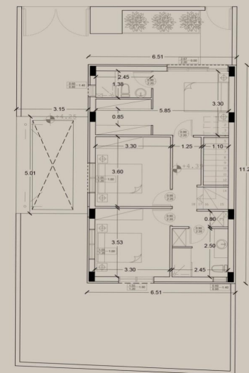
ΚΑΤΟΨΗ ΟΡΟΦΟΥ
