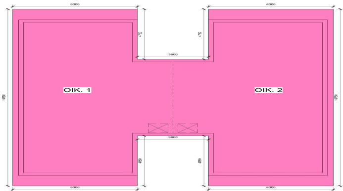
1 Οροφή - Ποσοστό Κάλυψης 1 : 100
