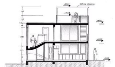
Τομη Α-Α
