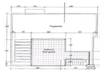
Ανοψη
