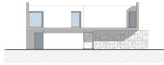
① ΟΨΗ 1 1 : 100
