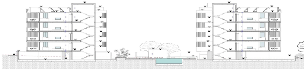
1 SITE SECTION 1:100
