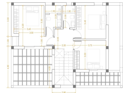
ΚΑΤΟΨΗ ΟΡΟΦΟΥ
