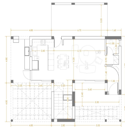
ΚΑΤΟΨΗ ΙΣΟΓΕΙΟ
