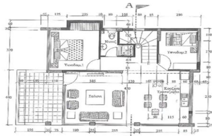
Κατοψη Ισογείου
