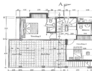
Κατοψη Οροφού
