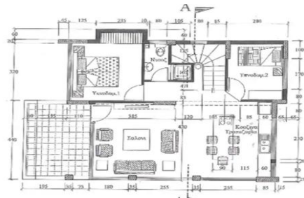
Κατοψη Ισογειου
