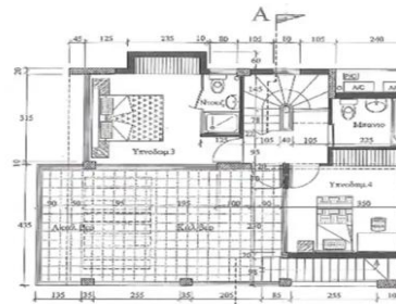
Κατοψη Οροφου
