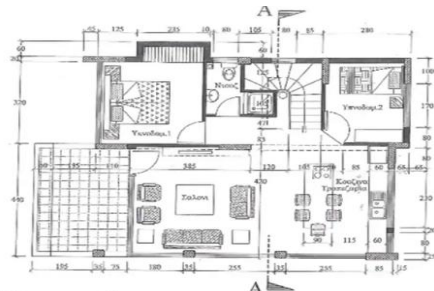
Κατοψη Ισογείου
