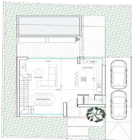
ΚΑΤΩΦΗ ΙΣΟΓΕΙΟΥ
