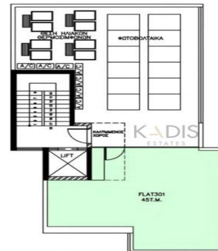
ΚΑΤΟΨΗ ΟΡΟΦΗΣ
