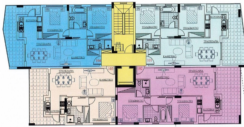
ΚΑΤΟΨΗ 1ου ΟΡΟΦΟΥ
