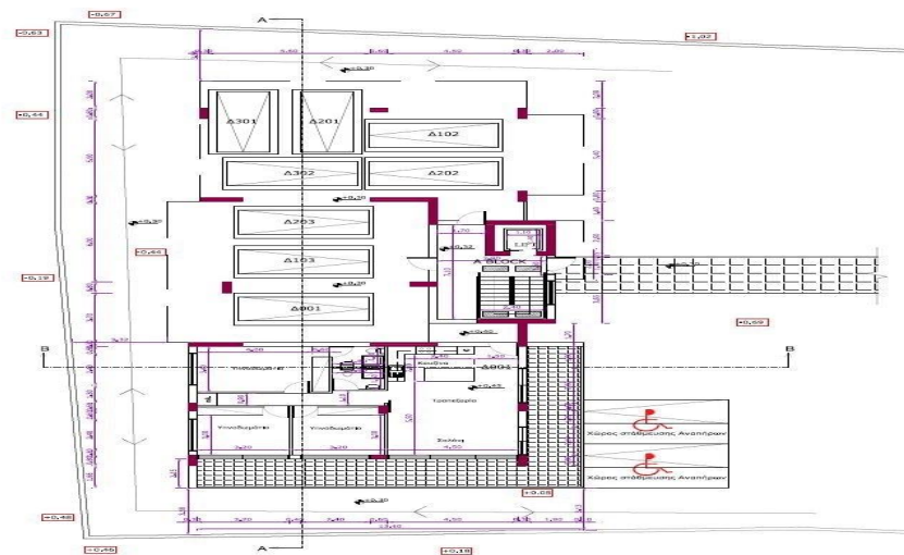
ΚΑΤΟΨΗ ΥΠΟΣΤΕΓΟΥ -BLOCK A
