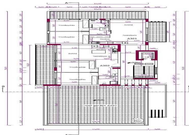
ΚΑΤΟΨΗ 3ου ΟΡΟΦΟΥ-BLOCK A
