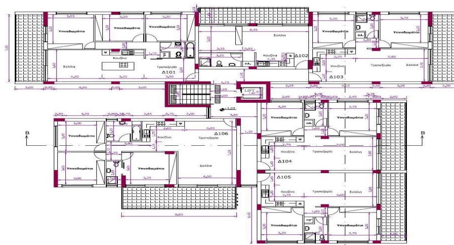
ΚΑΤΟΨΗ 1ου ΟΡΟΦΟΥ-BLOCK B
