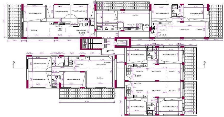
ΚΑΤΟΨΗ 1ου ΟΡΟΦΟΥ-BLOCK Β
