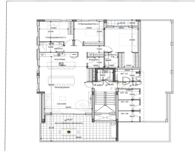
ΚΑΤΟΨΗ 2ου ΟΡΟΦΟΥ
