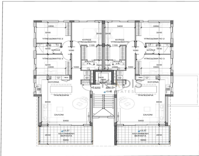
ΚΑΤΟΨΗ 1ου ΟΡΟΦΟΥ
