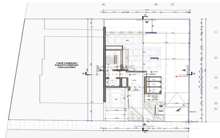
ΚΑΤΟΨΗ ΙΣΟΓΕΙΟΥ ΚΛΙΜΑΚΑ 1:200
