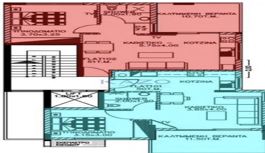
ΚΑΤΟΨΗ Α ΟΡΟΦΟΥ
