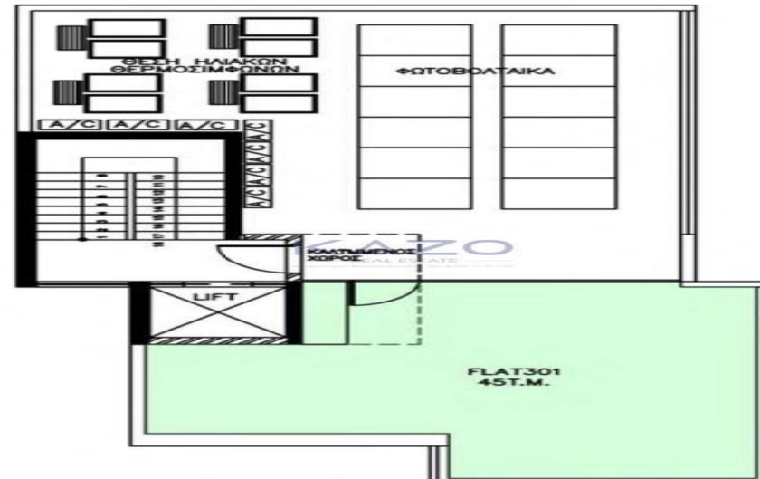
ΚΑΤΟΨΗ ΟΡΟΦΗΣ
