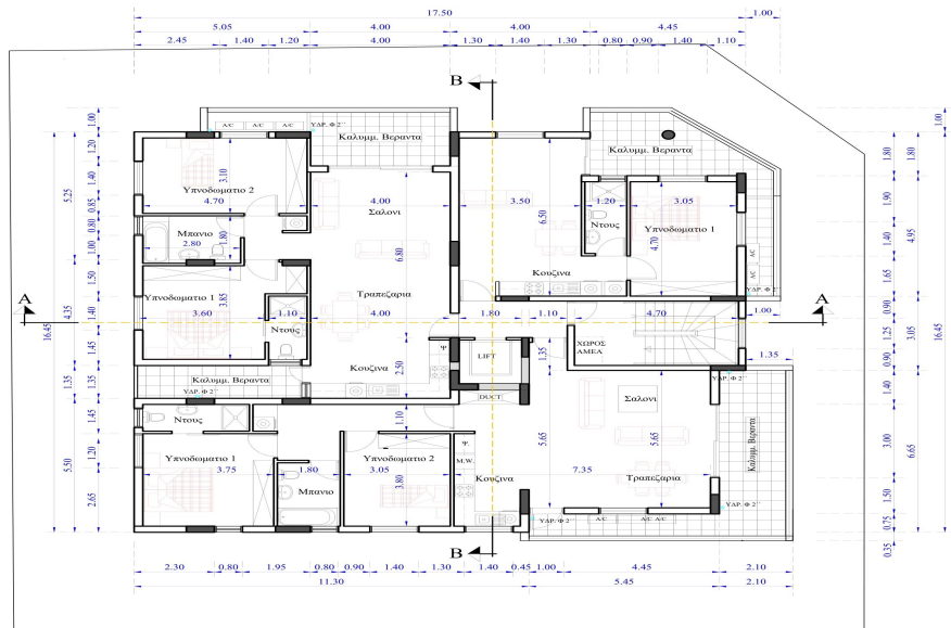
ΚΑΤΟΨΗ 2ου και 3ου ΟΡΟΦΟΥ
