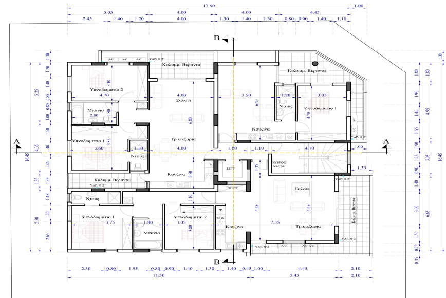
ΚΑΤΟΨΗ 1ου ΟΡΟΦΟΥ
