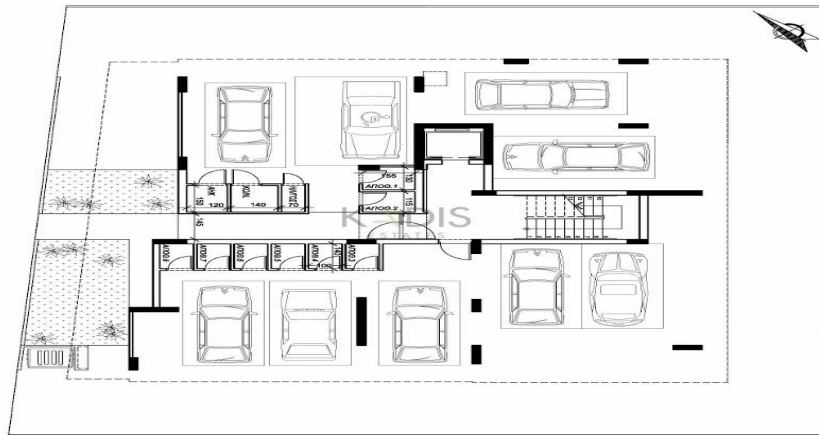
ΙΣΟΓΕΙΟ - ΠΥΛΩΤΗ
