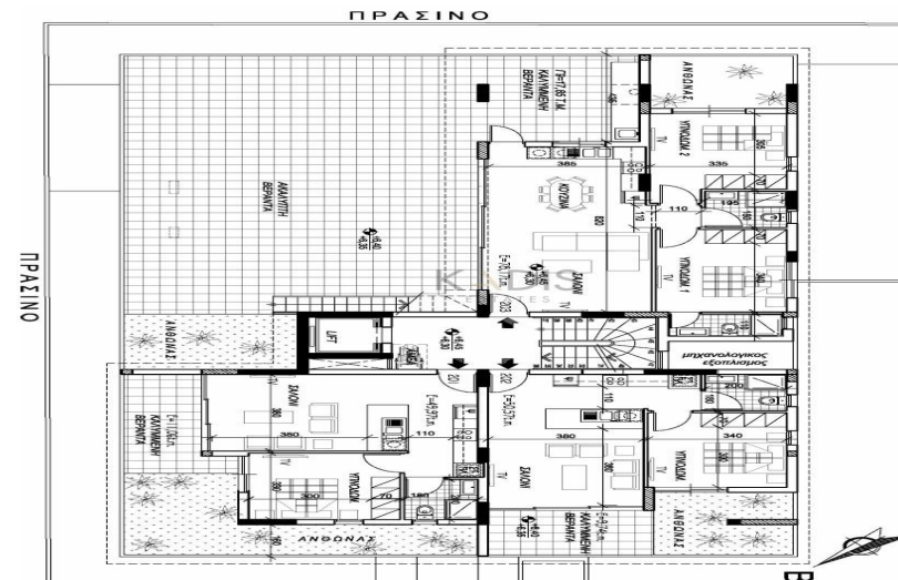
2 ος ΟΡΟΦΟΣ
