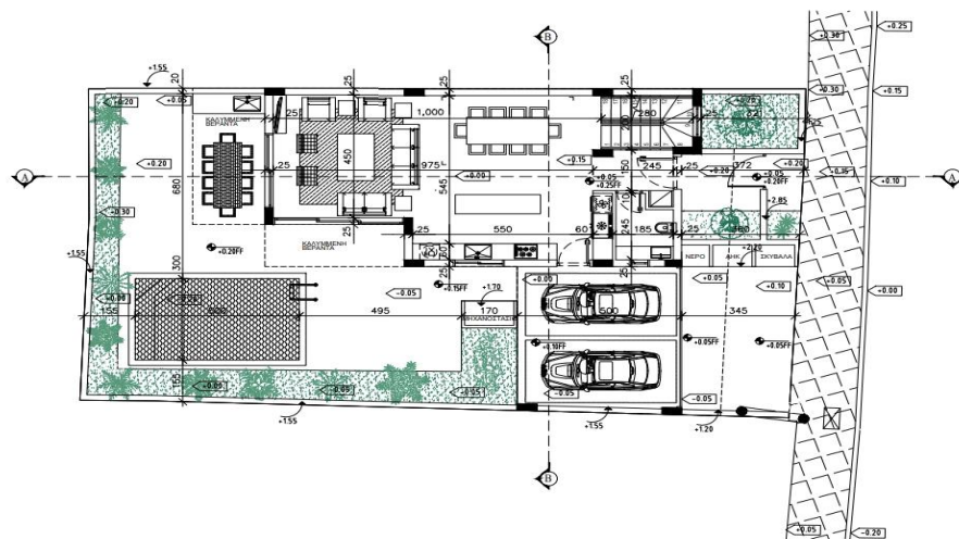
ΚΑΤΟΨΗ ΙΣΟΓΕΙΟΥ
