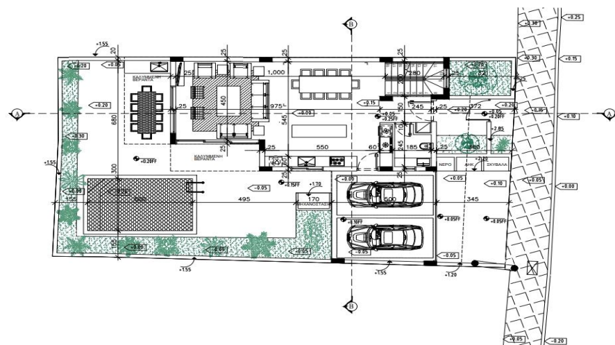
ΚΑΤΩΦΗ ΙΣΟΓΕΙΟΥ
