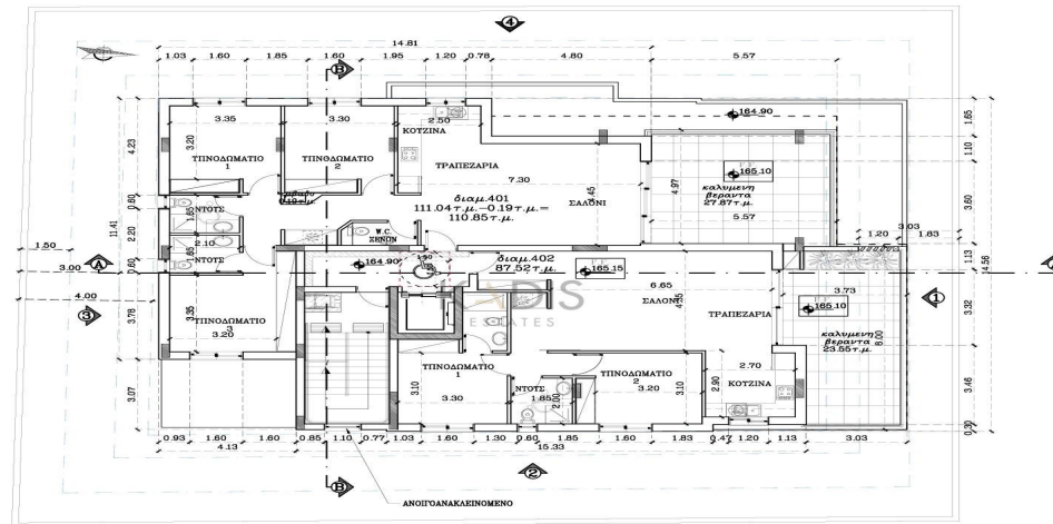
ΚΑΤΟΨΗ 4ου ΟΡΟΦΟΥ
