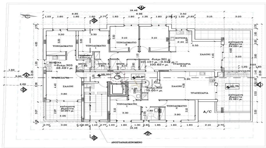
ΚΑΤΟΨΗ 3ου ΟΡΟΦΟΥ
