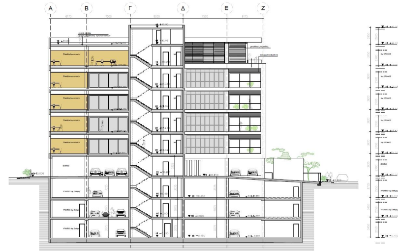
TOMH B-B' 1:200
