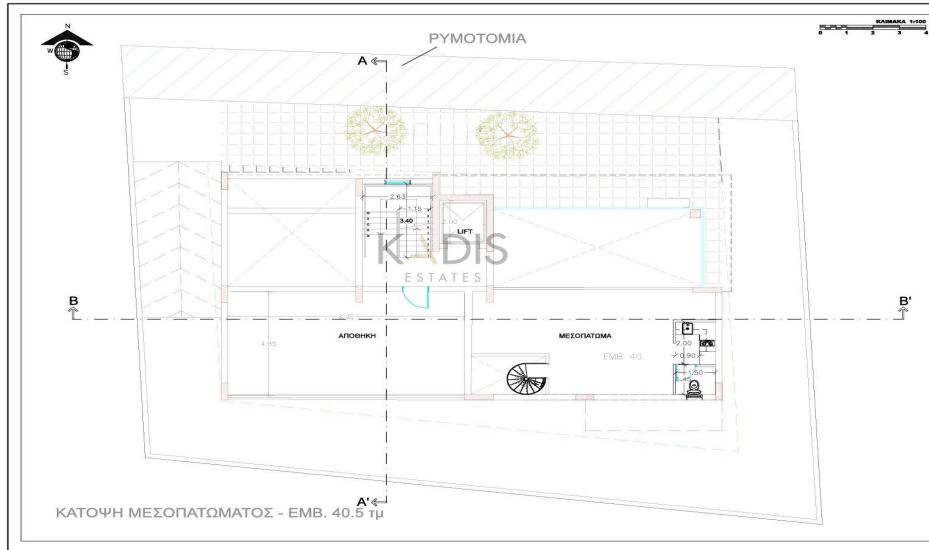
ΚΑΤΟΨΗ ΜΕΣΟΠΑΤΩΜΑΤΟΣ
