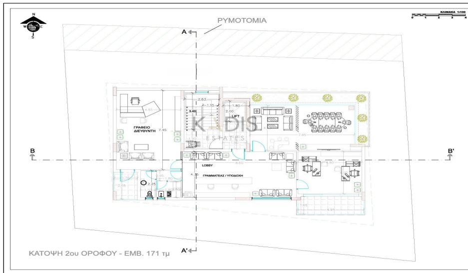
ΚΑΤΟΨΗ 2ου ΟΡΟΦΟΥ
