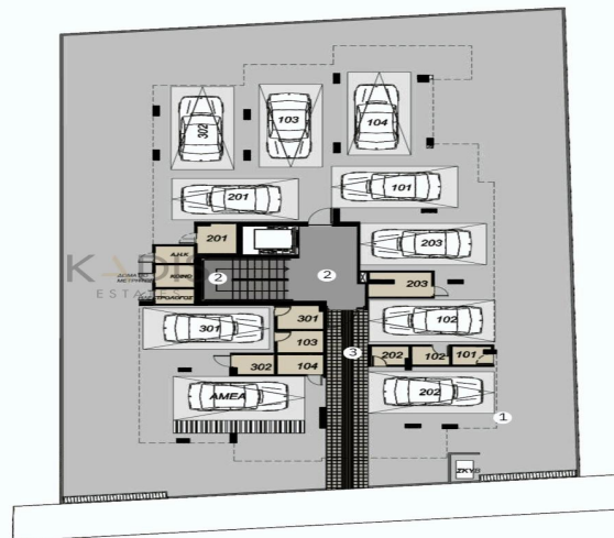
ΚΑΤΟΨΗ ΙΣΟΓΕΙΟΥ
