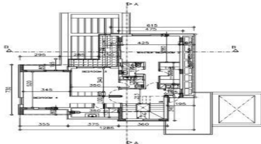
KATOHH OPOBOT KATOKIAS KAMAKA: 1:200
