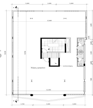
Κάτοψη τυπικού ορόφου (2ος & 3ος)
