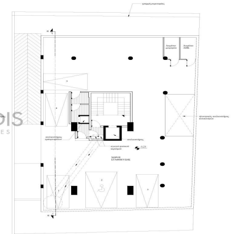
Κάτοψη ισόγειου (-1)
