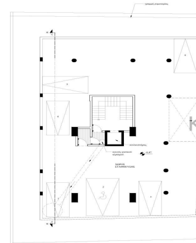
Κάτοψη ισόγειου (-2)
