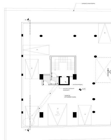
Κάτοψη ισόγειου (-2)
