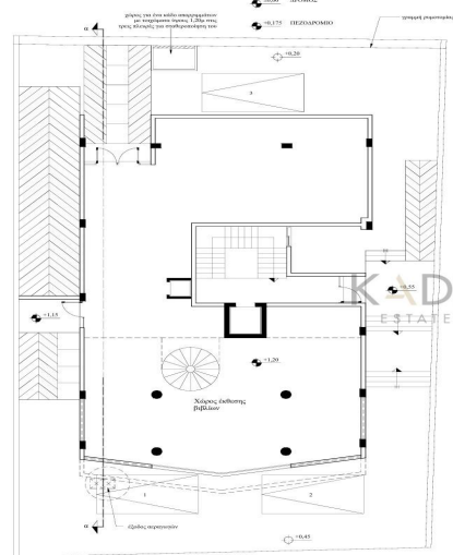
Κάτοψη ισόγειου
