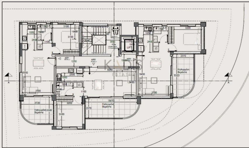
ΚΑΤΟΨΗ 2ΟΥ ΟΡΟΦΟΥ
