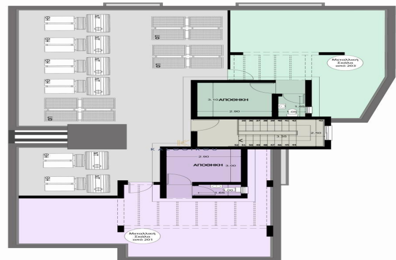
ΚΑΤΟΨΗ ΟΡΟΦΗΣ
