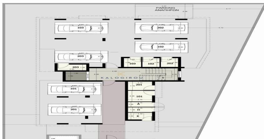
ΚΑΤΟΨΗ ΙΣΟΓΕΙΟΥ
