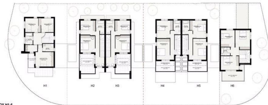
ΚΑΤΩΦΗ ΟΡΟΦΟΥ Η1-6 1:100
