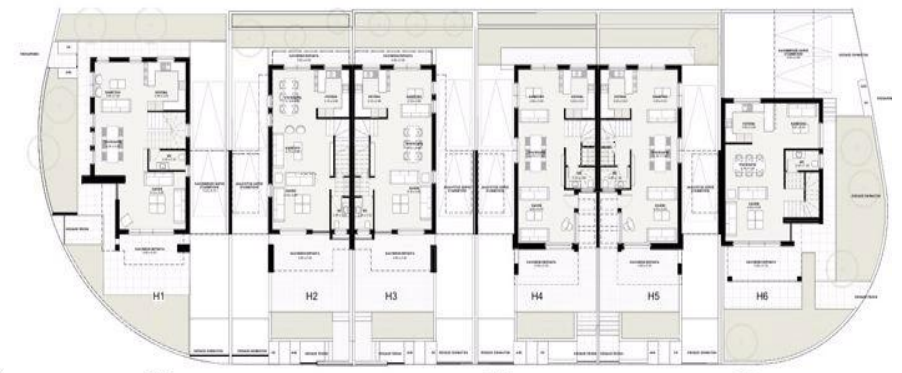
ΚΑΤΩΦΗ ΙΣΟΓΕΙΟΥ Η1-6 1:100
