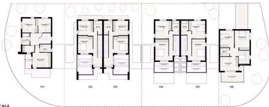
ΚΑΤΩΦΗ ΙΣΟΓΕΙΟΥ Η1-6 1:100
