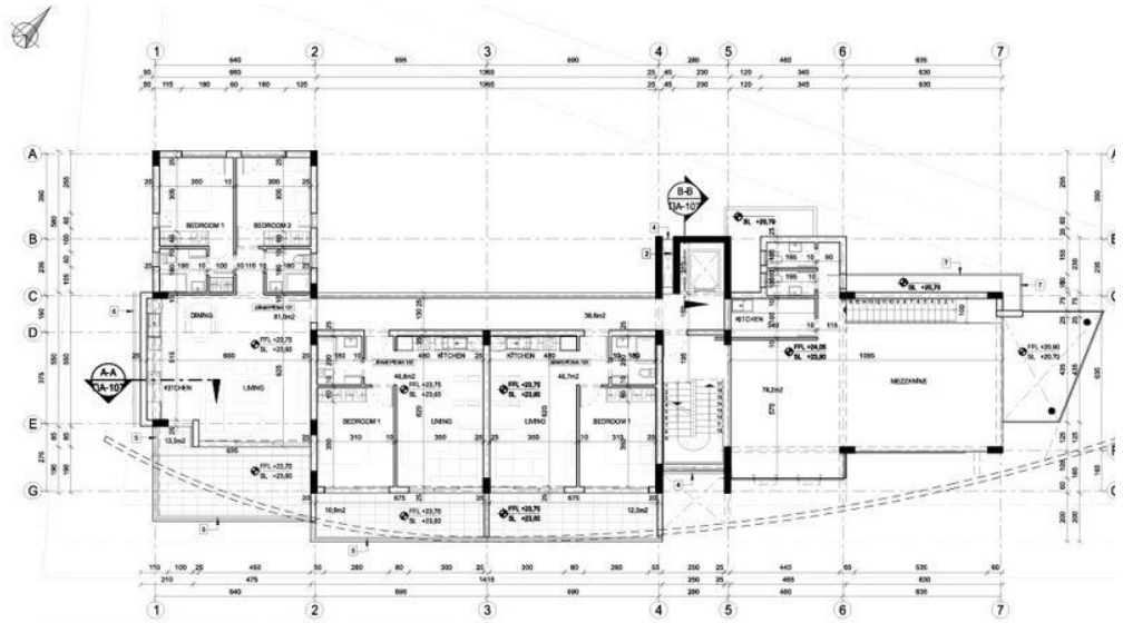
ΚΑΤΟΨΗ ΜΕΣΟΠΑΤΩΜΑΤΟΣ / 1ου ΟΡΟΦΟΥ
