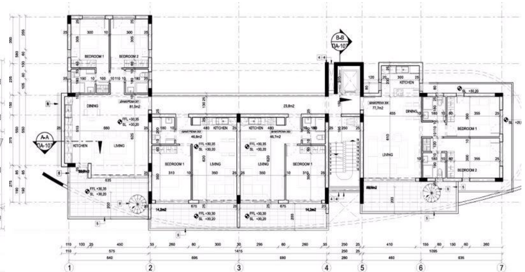
ΚΑΤΟΨΗ 3ου ΟΡΟΦΟΥ
