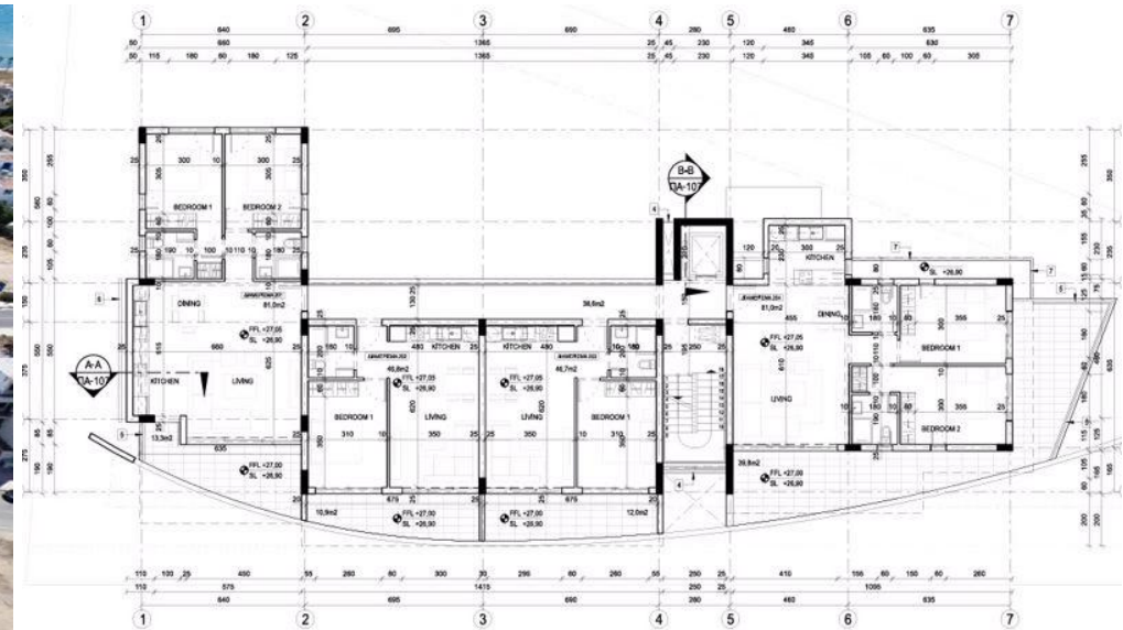
ΚΑΤΟΨΗ 2ου ΟΡΟΦΟΥ
