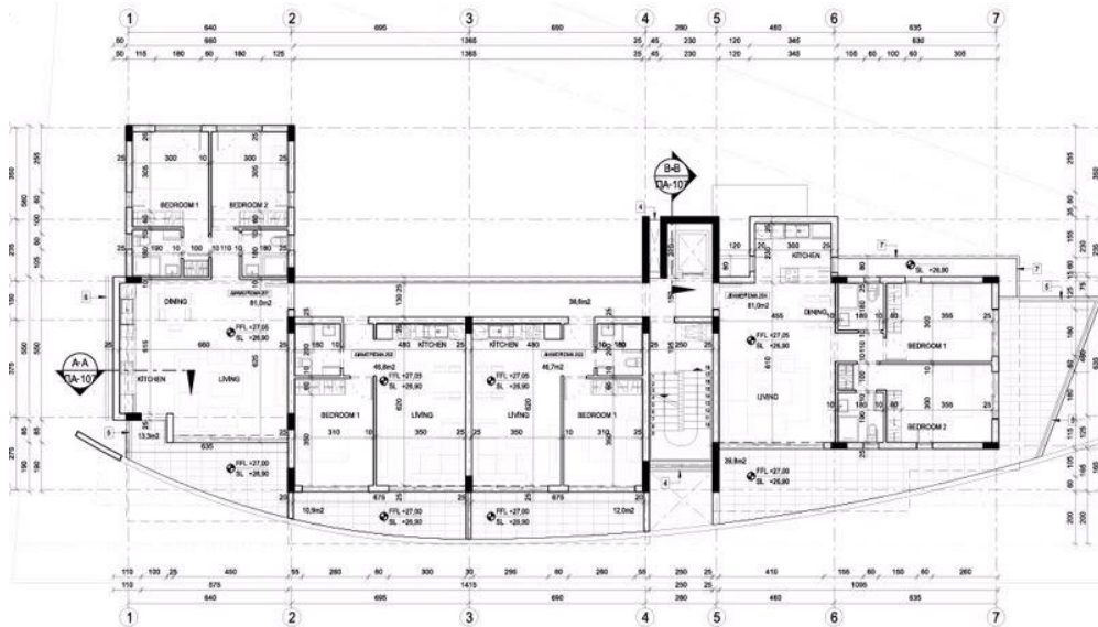
ΚΑΤΩΦΗ 2ου ΟΡΟΦΟΥ
