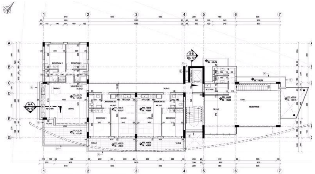
ΚΑΤΩΦΗ ΜΕΣΟΠΑΤΩΜΑΤΟΣ / 1ου ΟΡΟΦΟΥ
