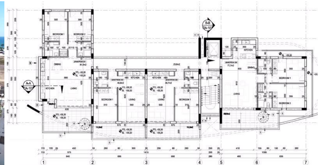
ΚΑΤΩΦ 3ου ΟΡΟΦΟΥ
