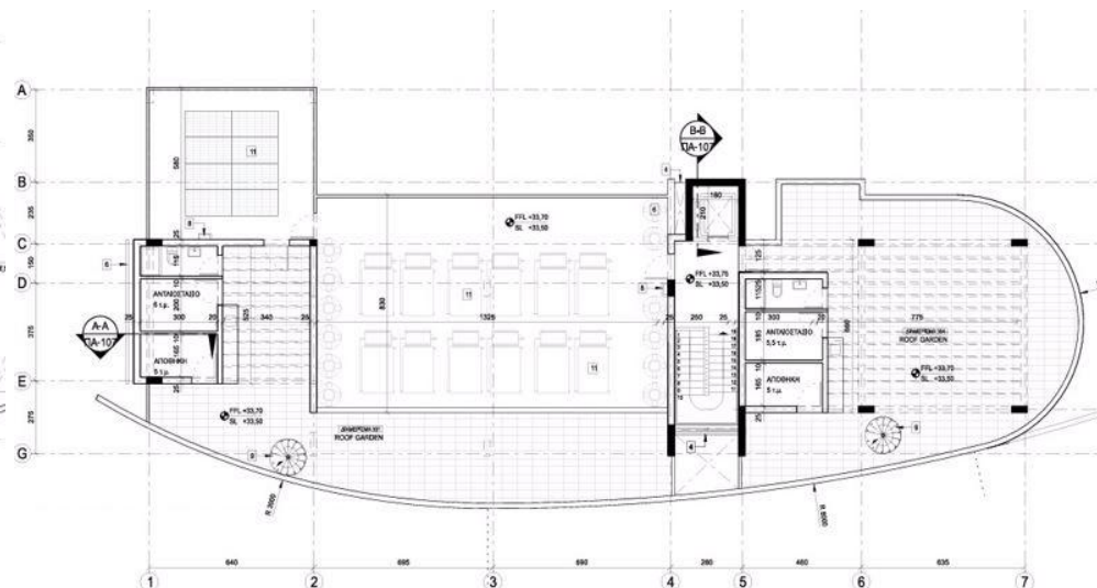
ΚΑΤΟΨΗ ΟΡΟΦΗΣ
