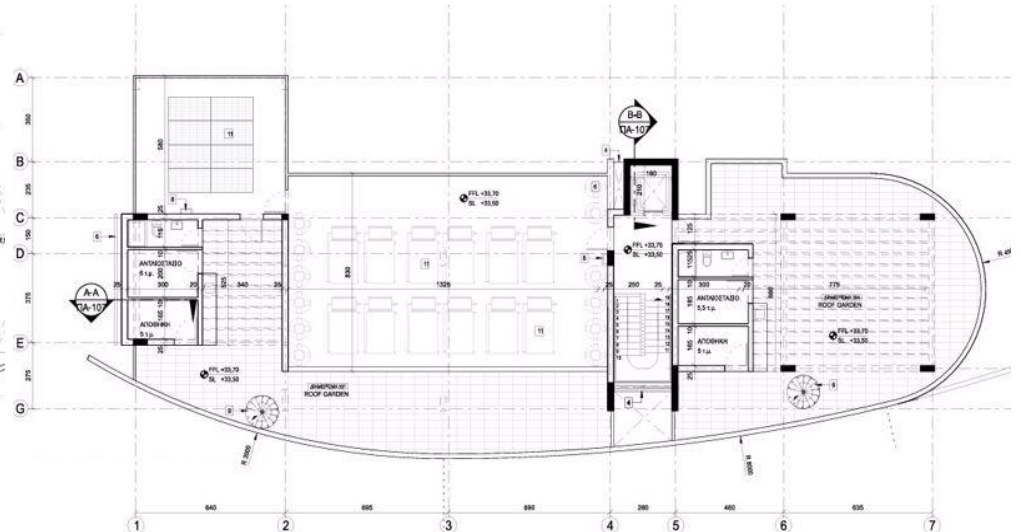
ΚΑΤΟΨΗ ΟΡΟΦΗΣ
