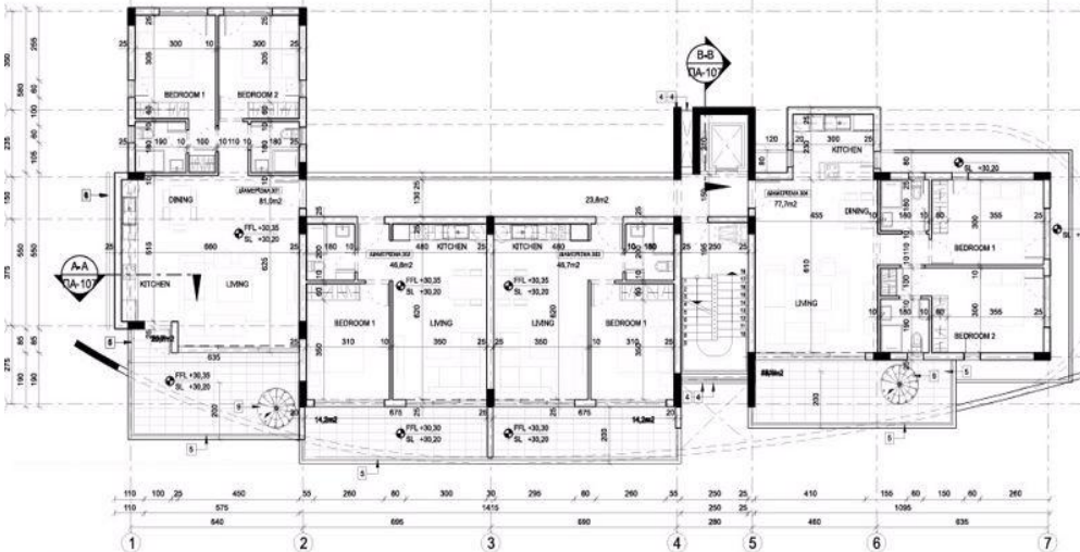
ΚΑΤΟΨΗ 3ου ΟΡΟΦΟΥ
