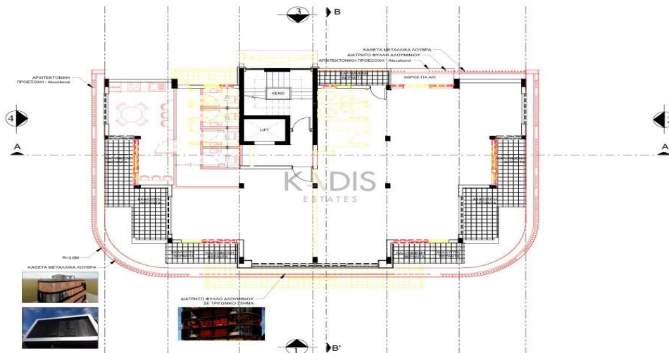
ΠΡΟΣΘΗΚΟΜΕΤΑΤΡΟΠΕΣ - ΚΑΤΟΠΗ 1ου ΟΡΟΦΟΥ Κλίμακα 1:100
