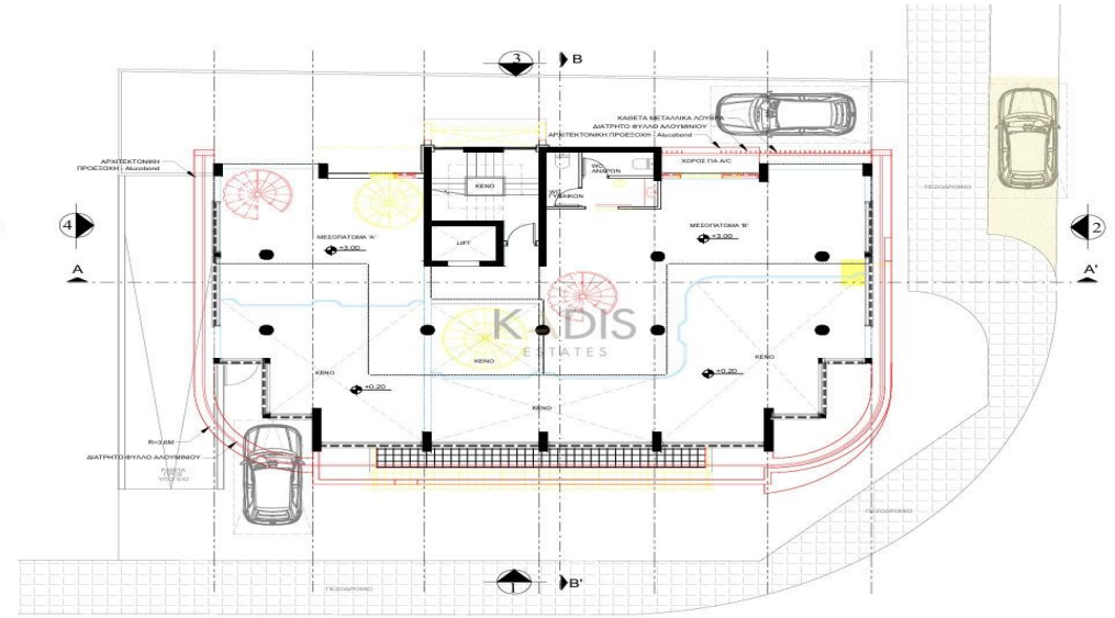
ΠΡΟΣΘΗΚΟΜΕΤΑΤΡΟΠΕΣ - ΚΑΤΟΠΗ ΜΕΣΟΠΑΤΩΜΑΤΟΣ Κλίμακα 1:100
