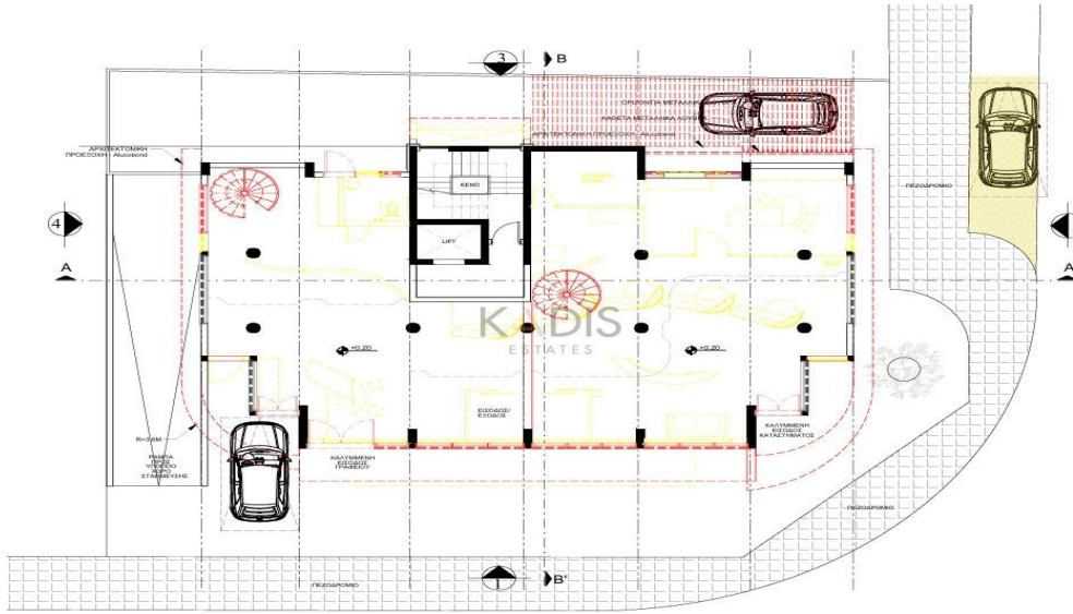
ΠΡΟΣΘΗΚΟΜΕΤΑΤΡΟΠΕΣ - ΚΑΤΟΨΗ ΙΣΟΓΕΙΟΥ Κλίμακα 1:100
