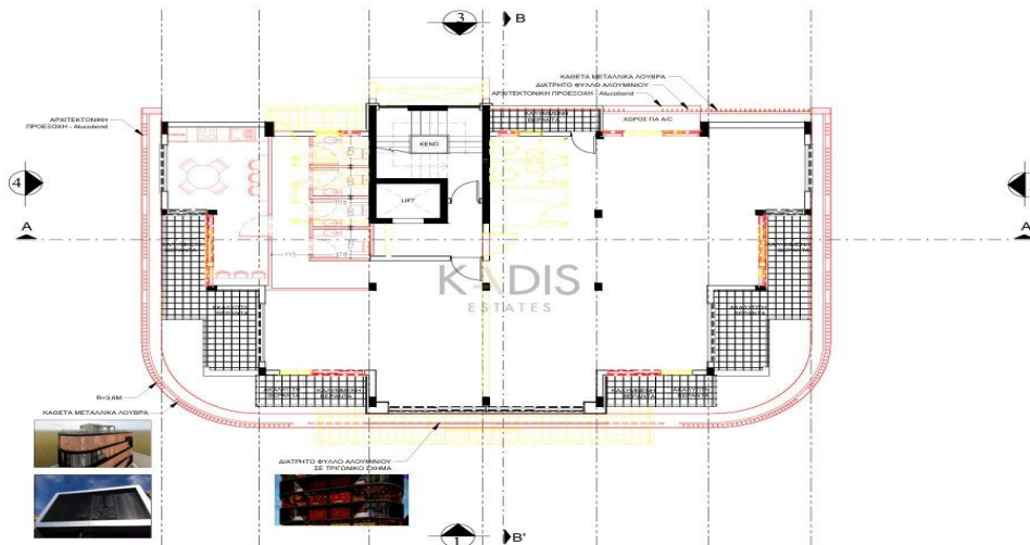
ΠΡΟΣΘΗΚΟΜΕΤΑΤΡΟΠΕΣ - ΚΑΤΟΨΗ 1ου ΟΡΟΦΟΥ Κλίμακα 1:100
