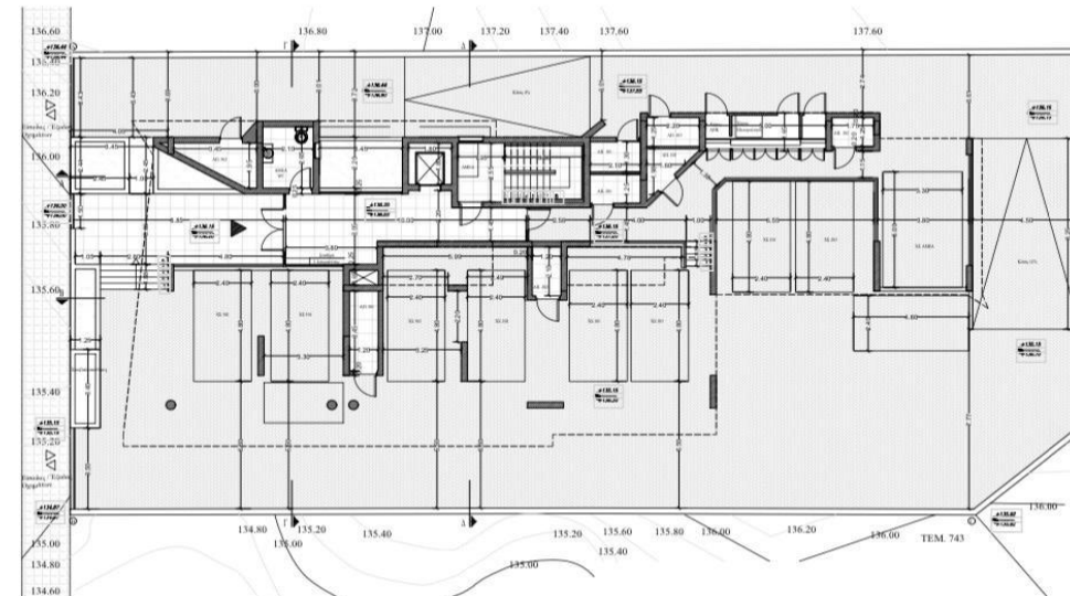
Κάτοψη Ισογείου
