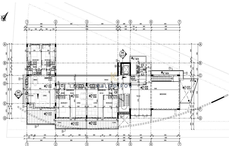
ΚΑΤΟΨΗ ΜΕΣΟΠΛΩΜΑΤΟΣ / 1ου ΟΡΟΦΟΥ
