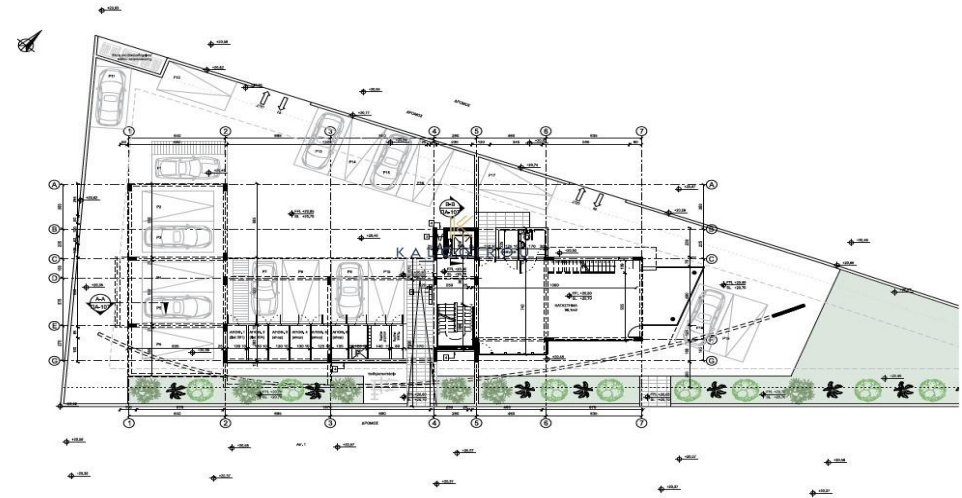
ΚΑΤΟΨΗ ΙΣΟΓΕΙΟΥ
