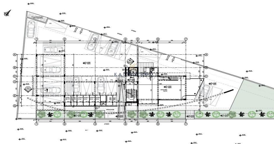
ΚΑΤΟΨΗ ΙΣΟΓΕΙΟΥ
