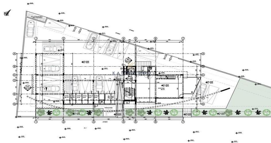
ΚΑΤΟΨΗ ΙΣΟΓΕΙΟΥ
