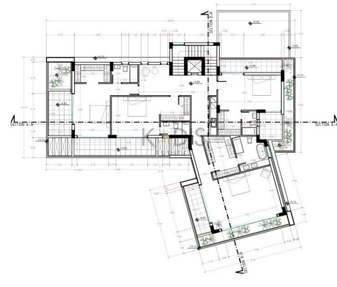
ΚΑΤΩΦΗ ΟΡΟΦΟΥ
