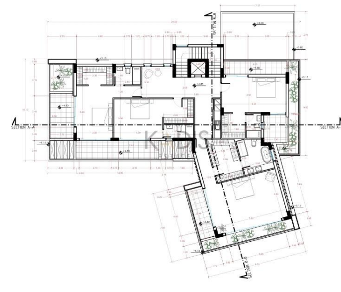
ΚΑΤΩΦΗ ΟΡΟΦΟΥ
