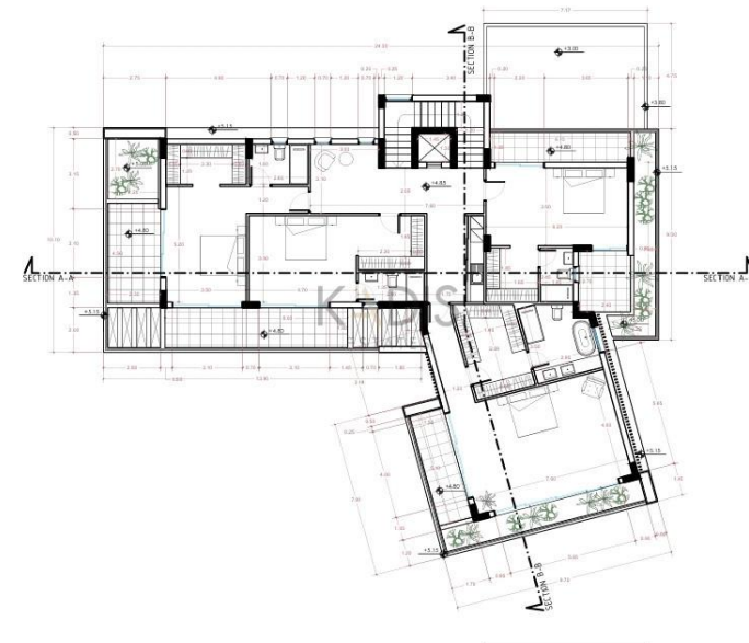
ΚΑΤΩΦΗ ΟΡΟΦΟΥ
