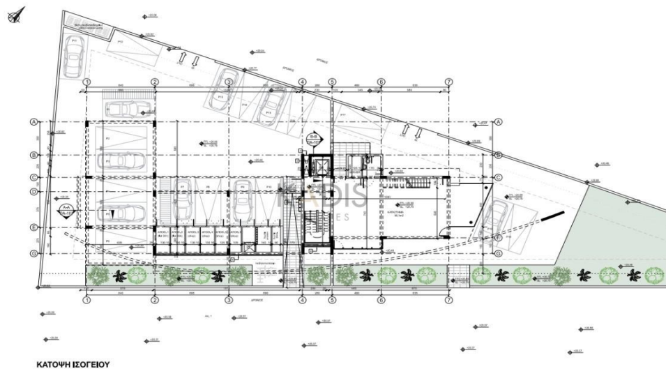
ΚΑΤΟΨΗ ΙΣΟΓΕΙΟΥ
